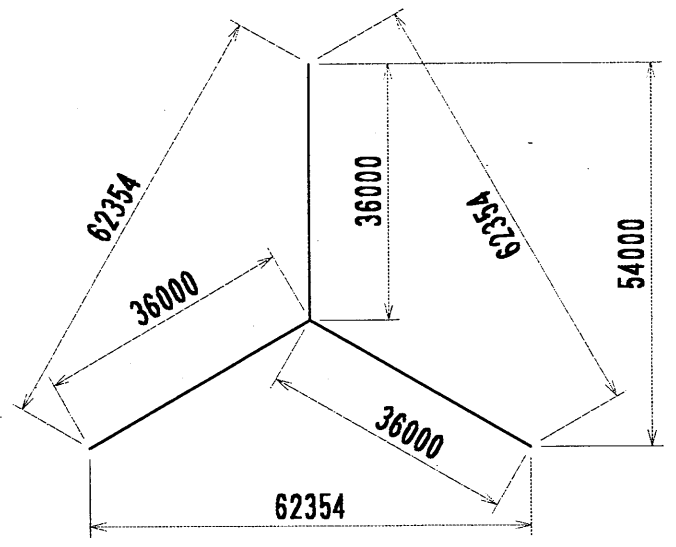
アンカー位置詳細図
